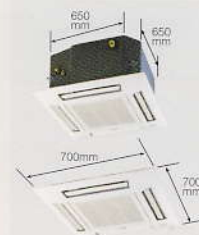
Panel: CZ-BT20E
